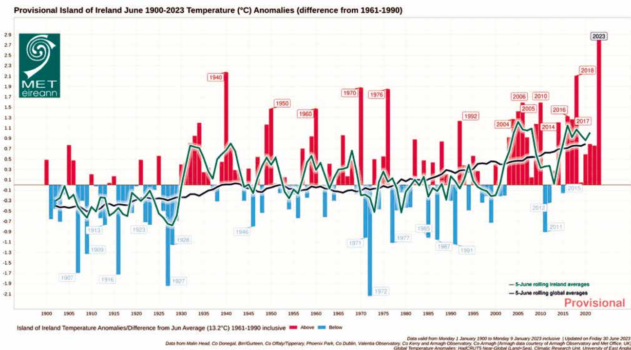
Fíor 1.1: Éire 1900 – 2023 Neamhréireanna Teochta (°C), Ráiteas Bliantúil Aeráide d'Éirinn 2023 (Met Éireann)
