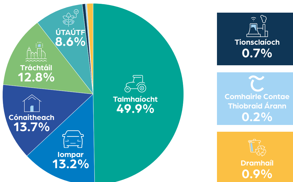
Fíor 4.3: Astaíochtaí CO 2 eq in aghaidh na hEarnála i gContae Thiobraid Árann, 2018
