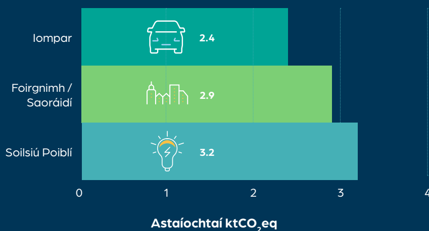
Fíor 4.5: Miondealú ar astaíochtaí GCT 2018 in ktCO 2 eq ag an gComhairle – roinnte de réir catagóire úsáide suntasach fuinnimh
