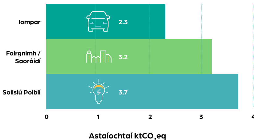
Fíor 4.6: Miondealú ar astaíochtaí GCT 2016 – 2018 i ktCO 2 eq ag an gComhairle – roinnte de réir catagóire úsáide suntasach fuinnimh
